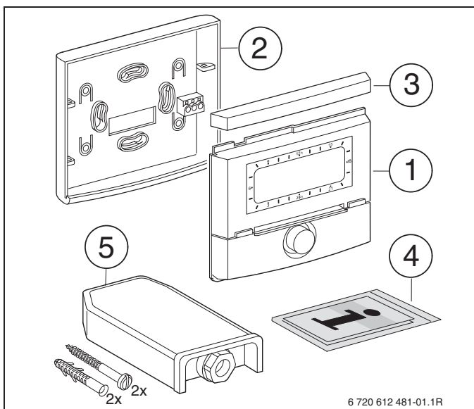
Sl. 2 Opis dobavljene opreme
