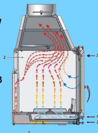
1. Zrak za izgorevanje lesa 2. Zrak za emisije po izgorevanju 3. Zrak za čiščenje stekla
